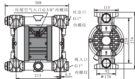
PP、PVDF、铝合金 (单位: mm)
