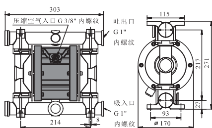
不锈钢316 (单位: mm)
